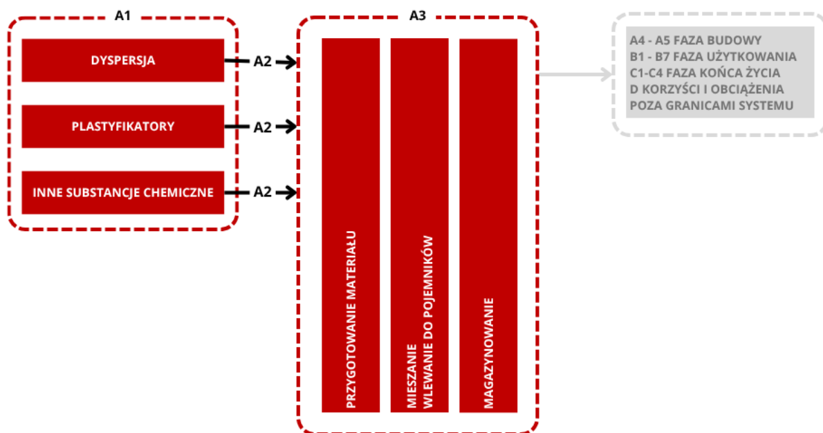
Rysunek 5.1: Granice systemu dla charakterystyki środowiskowej farb ogniochronnych
